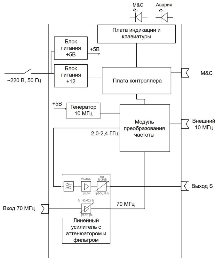
Рисунок 2 – Структурно-функциональная схема ПЧ «вверх»
