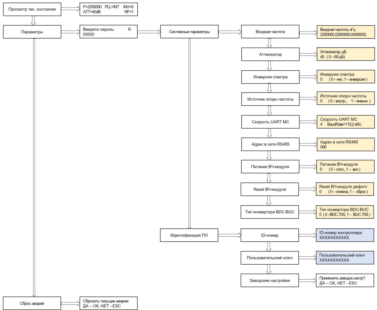
Рисунок 3 – Дерево меню ПЧ «вверх»
